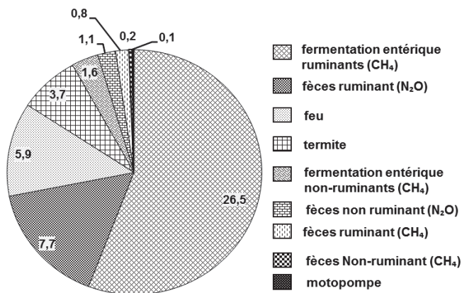
Figure 4 : Principales sources d'émission de GES (en kt eq.CO 2 /an)
