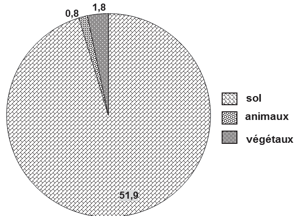
Figure 3 : Accumulation de carbone dans les principaux stocks de l'écosystème sylvo-pastoral (en kt eq.CO 2 /an)
