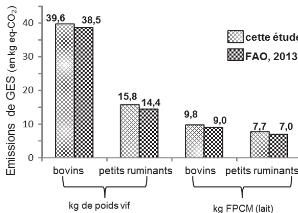
Figure 5 : Bilans GES brut par kg de produits animaux et par espèce
