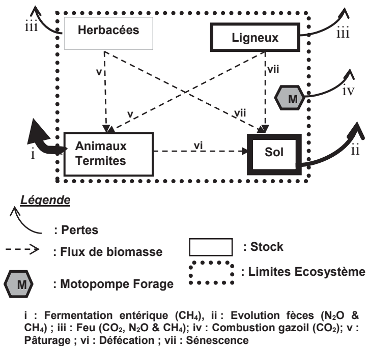
Figure 1 : Modèle conceptuel simplifié du fonctionnement d'un écosystème sylvo-pastoral en terme de stock-flux de carbone et azote.
