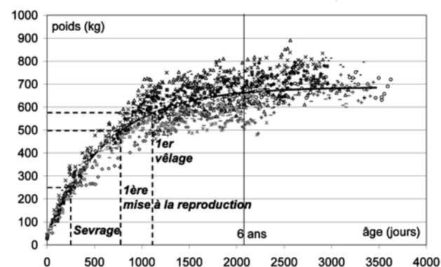
Figure 1 : croissances (21 vaches) et courbe moyenne calculée
